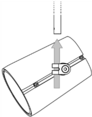
Etape E : Raccrochage sur perchoir
