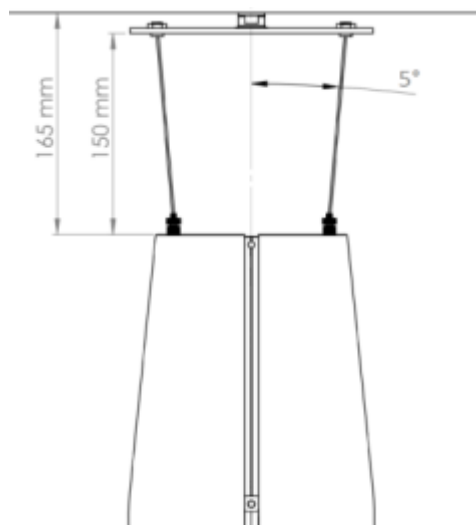
Distance minimale entre arrière d'une enceinte AS-5 et plafond de support de suspension : 165 mm
